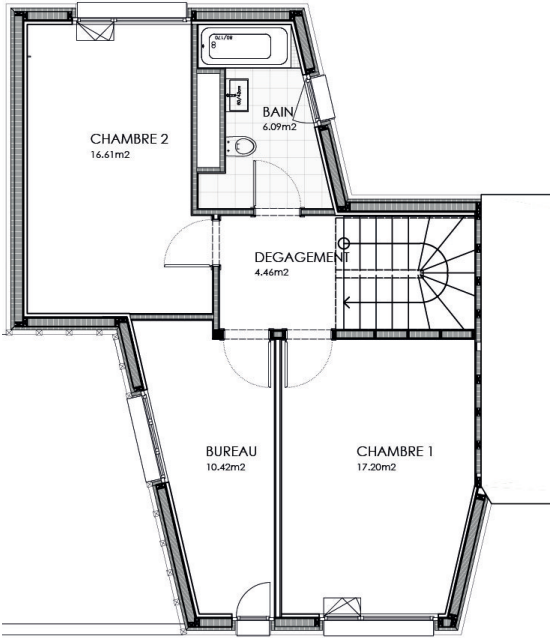
1er étage
